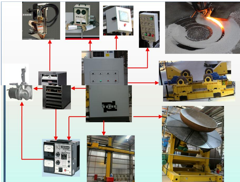
图 3：带极堆焊的组成
