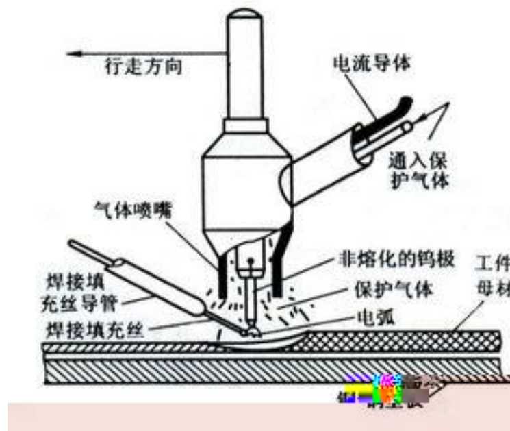
图 1 非熔化极氩弧焊的工作原理
